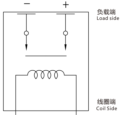
原理图 Schematic Diagram
