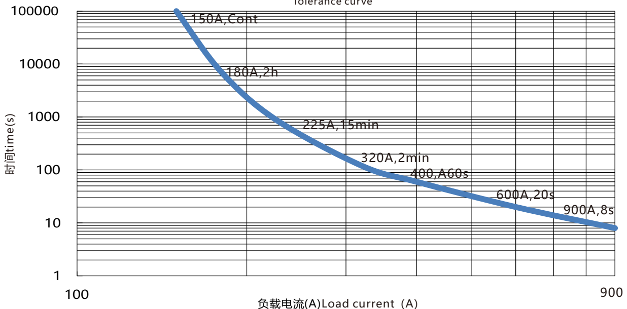
耐受能力曲线图 Tolerance curve
